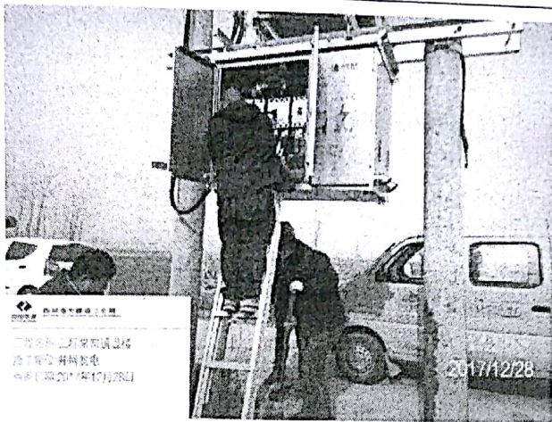
三标汴岗镇安装汇流箱计量柜
