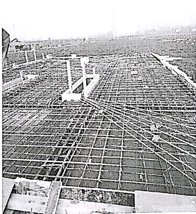
光伏区箱逆变基础钢筋绑扎
