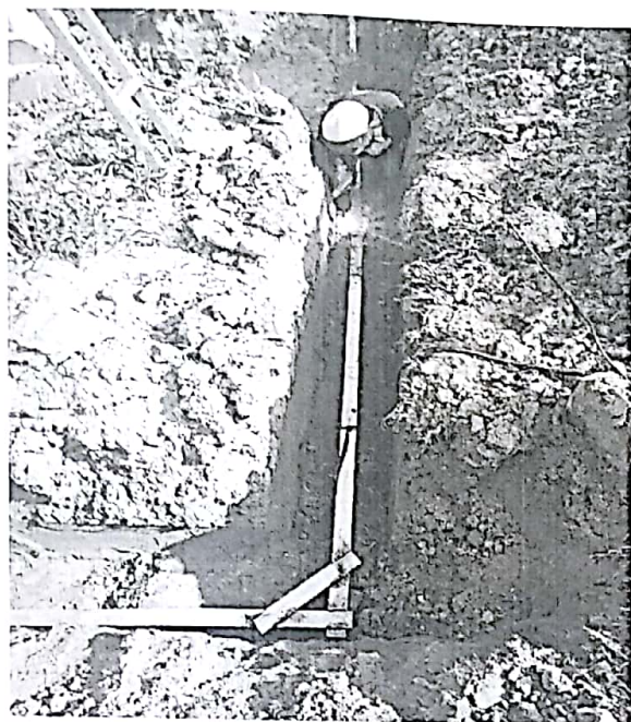
光伏区接地焊接
