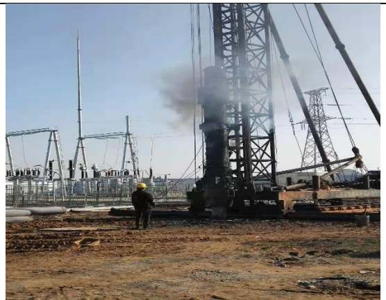
综合楼基础打桩施工
