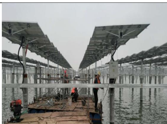
光伏区组件安装
