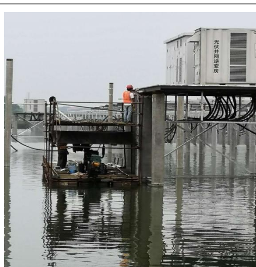
现场箱逆变平台加固焊接
