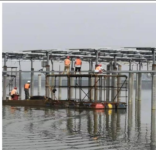
光伏区电缆敷设
