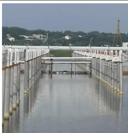
光伏区桥架安装
