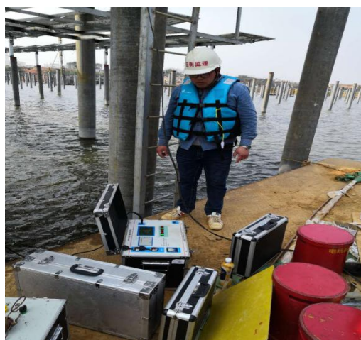
对现场耐压试验旁站
