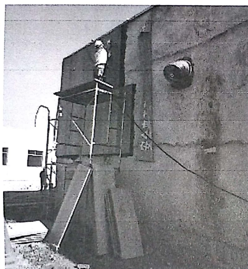
配电楼外墙保温施工
