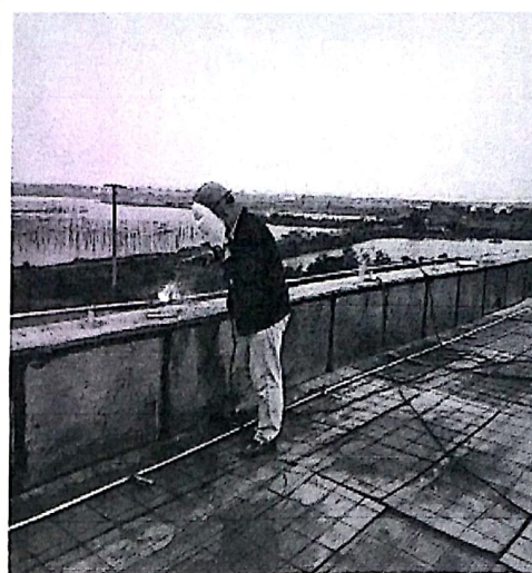
办公楼屋面避雷网施工
