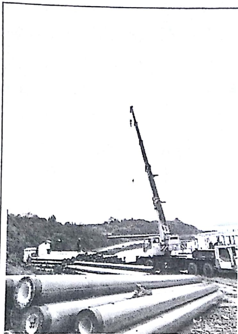
光伏区管桩吊运
