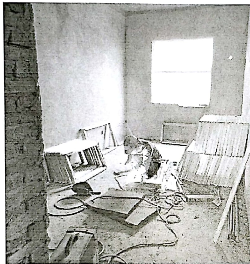
电缆沟盖板角铁外框制作
