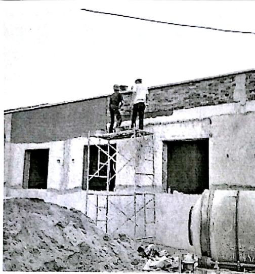
办公楼外墙抹灰施工
