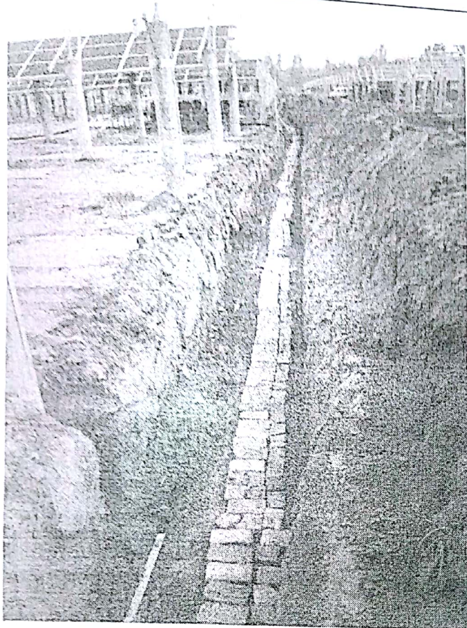
电缆铺砂盖砖
