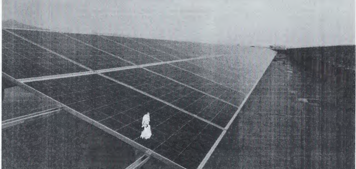
瑞金市“十二五”贫困村光伏扶贫扩面工程 乐群塑胶厂房屋顶光伏组件20181120
