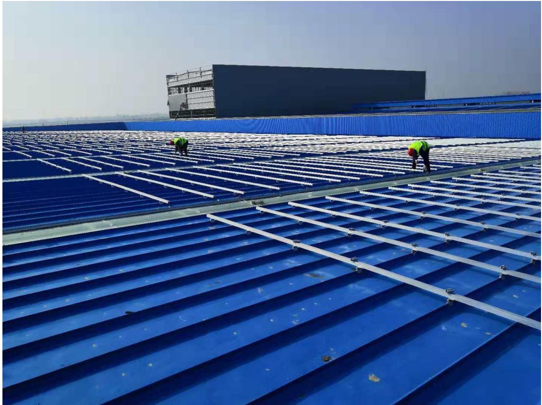
皮阿诺 D 号厂房压块、檩条安装
