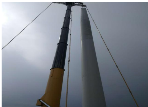
B08 号机位塔筒吊装
