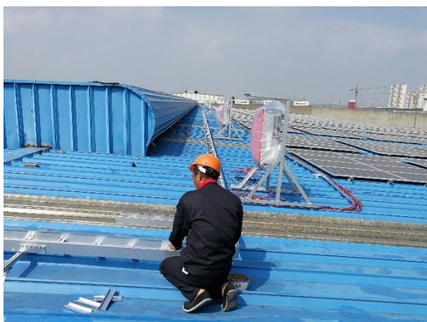
桥架安装
