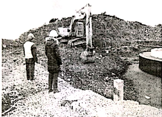
18#风机基础土方机械回填、夯实
