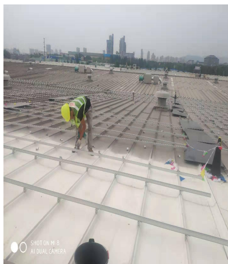
1 期厂房屋面支架安装
