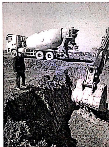
开关站基础垫层浇筑
