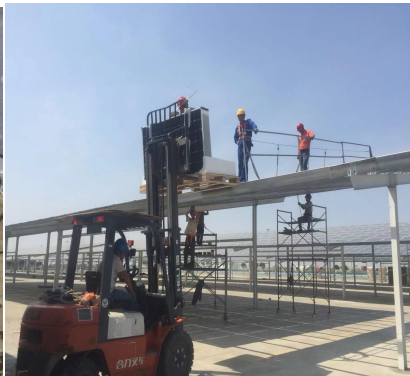
组件安装
