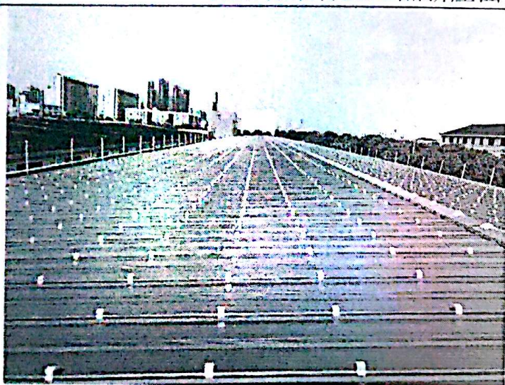
兄弟标准件施工点新屋面安全护网安装完成
