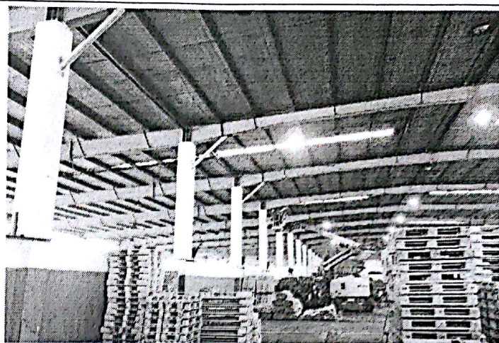
兄弟 2#屋面斜撑加固
