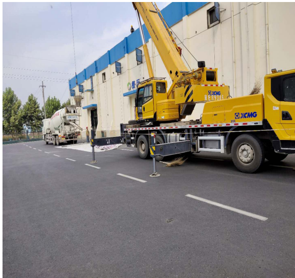
混凝土吊运
