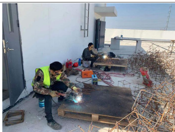
钢筋笼焊接
