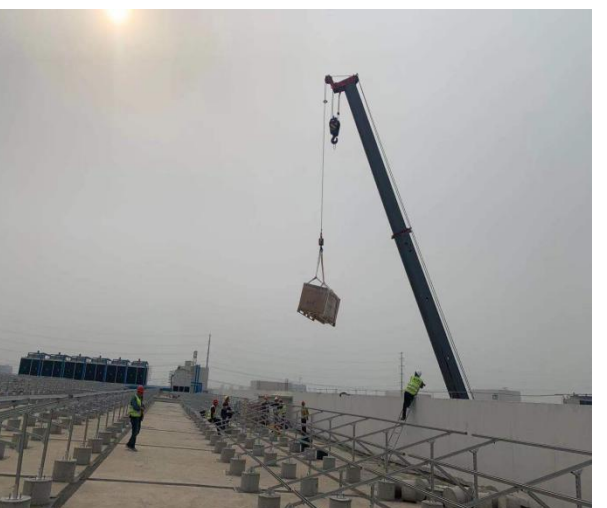
吊装组件
