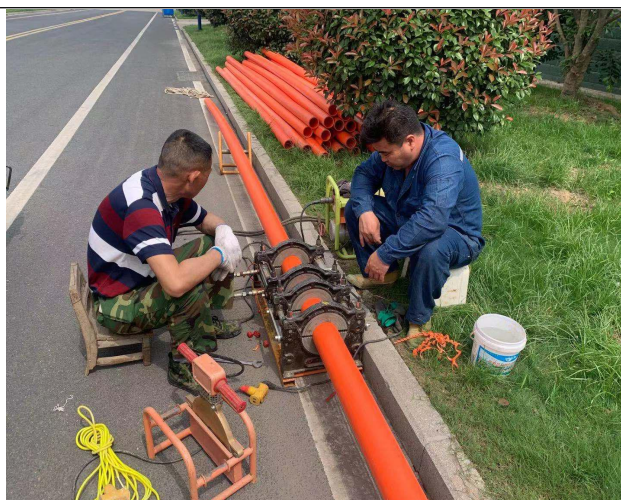
顶管熔接
