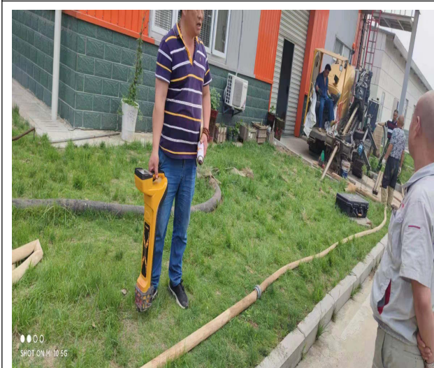
顶管施工
