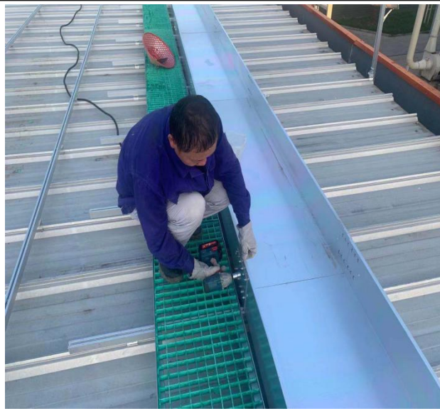
桥架安装
