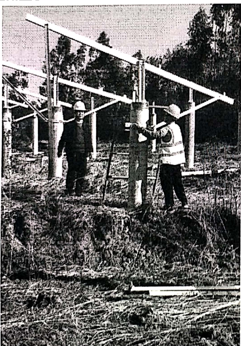
22#区支架安装检查
