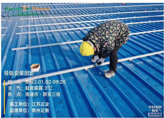
导轨安装固定
