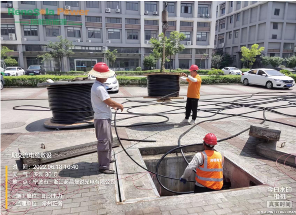
交流电缆敷设
