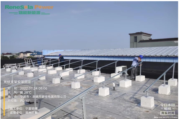
光伏支架安装固定
