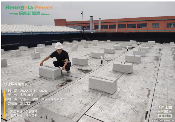
水泥墩间距检查
