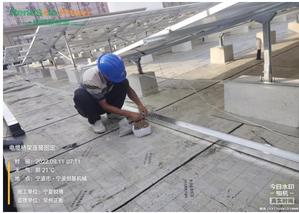
电缆桥架分散连接
