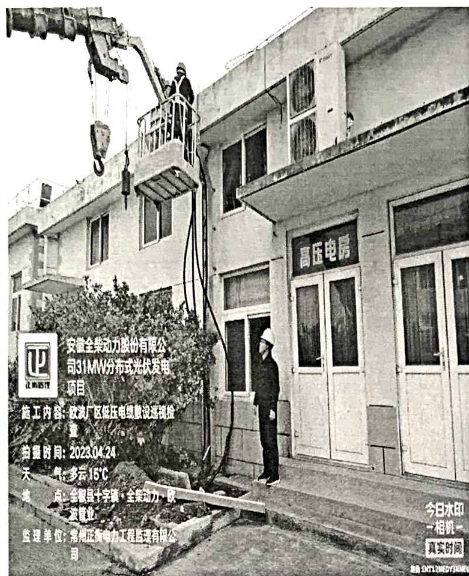
欧波厂区低压电缆敷设巡视检查
