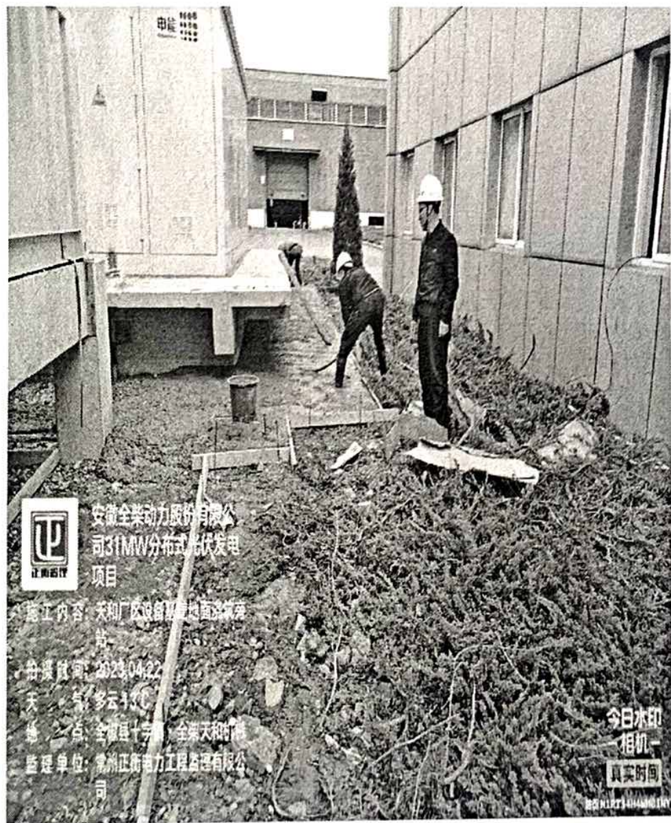
天和厂区基础基础地面浇筑旁站
