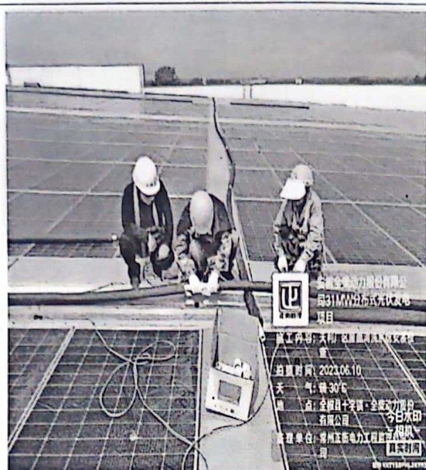
天利厂区屋面清洗系统安装检查
