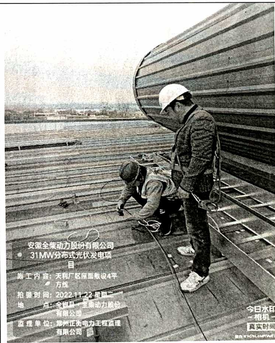
天利直流电缆敷设检查
