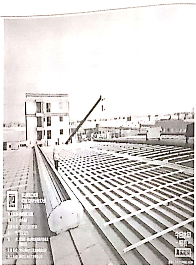
组件吊装
