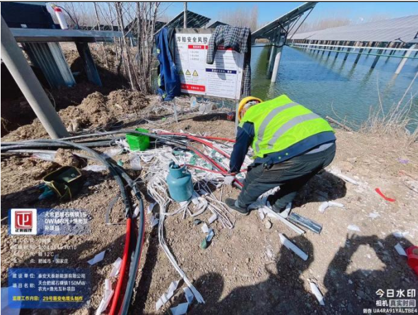
箱变一体机低压电缆头制作
