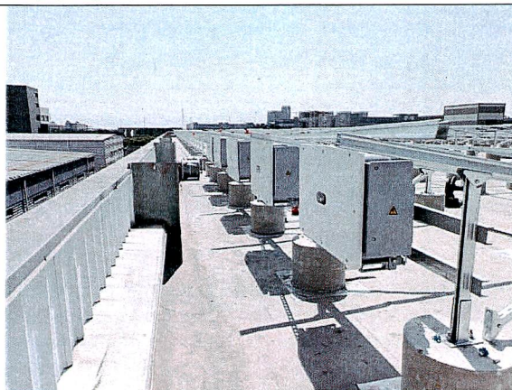
逆变器安装
