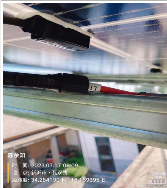
接地电阻测试
