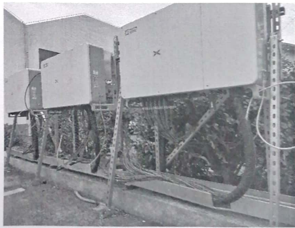
逆变器接线
