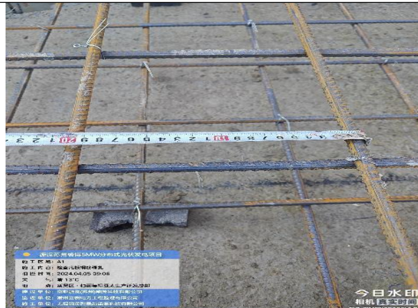
检查底板钢筋绑扎
