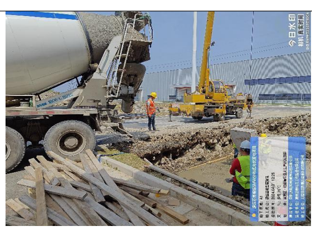
设备基础垫层浇筑
