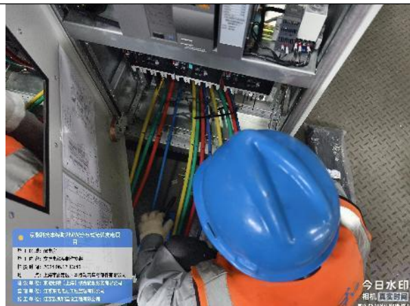
组件接地线安装
