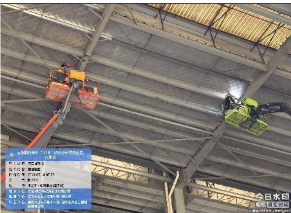
联合厂房主车间加固
