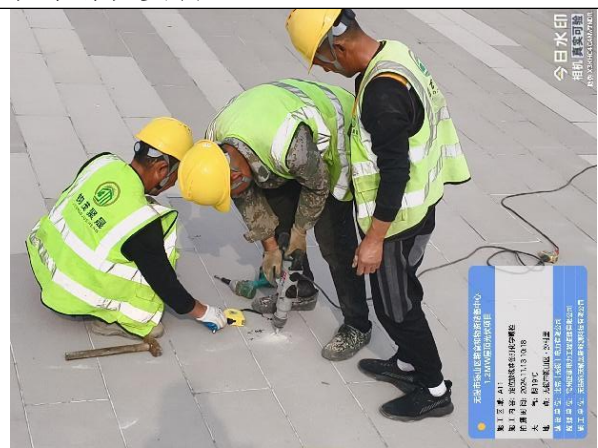
化学螺栓安装
