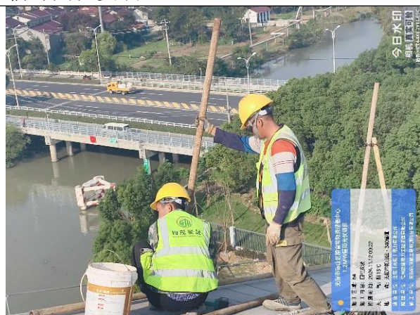
化学螺栓、TPO支架进场安装
