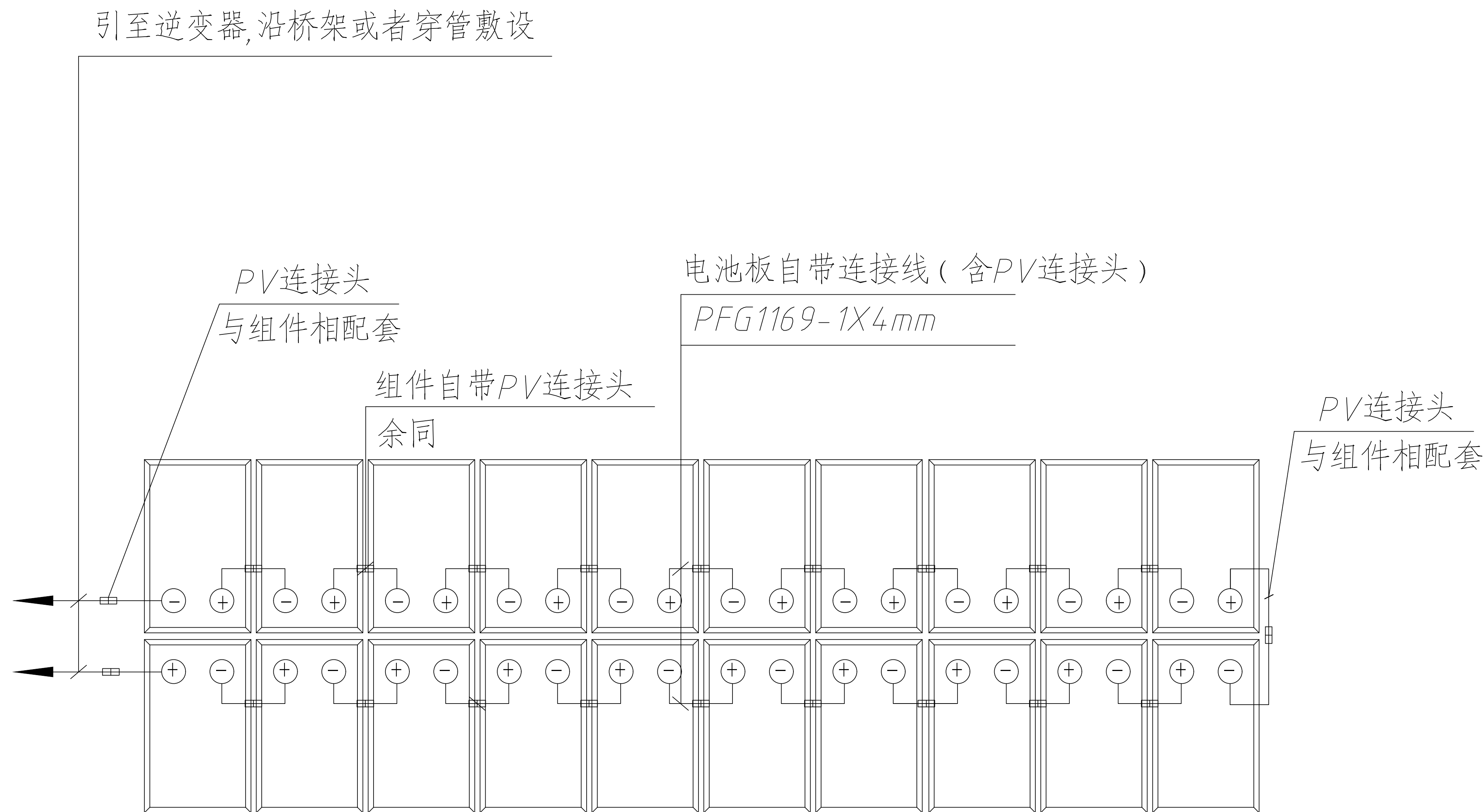
阵列组串电气接线图
