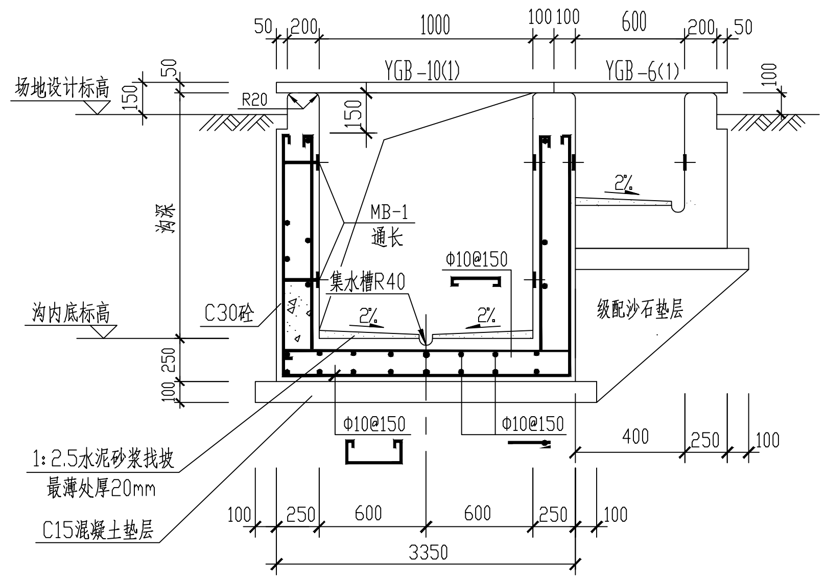
一般地段电缆沟断面图（二）
