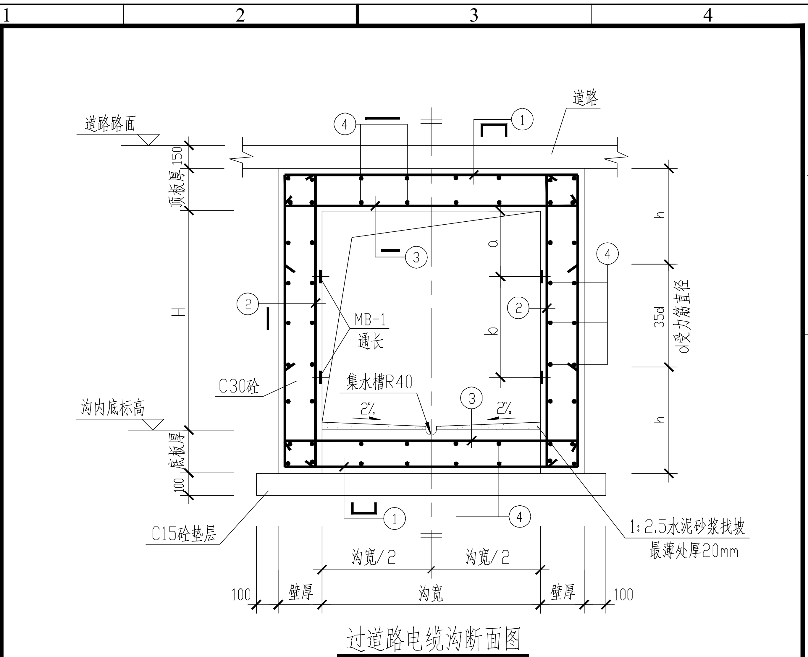
过道路电缆沟截面及配筋一览表
