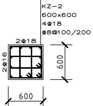
框架柱配筋图 1:50
