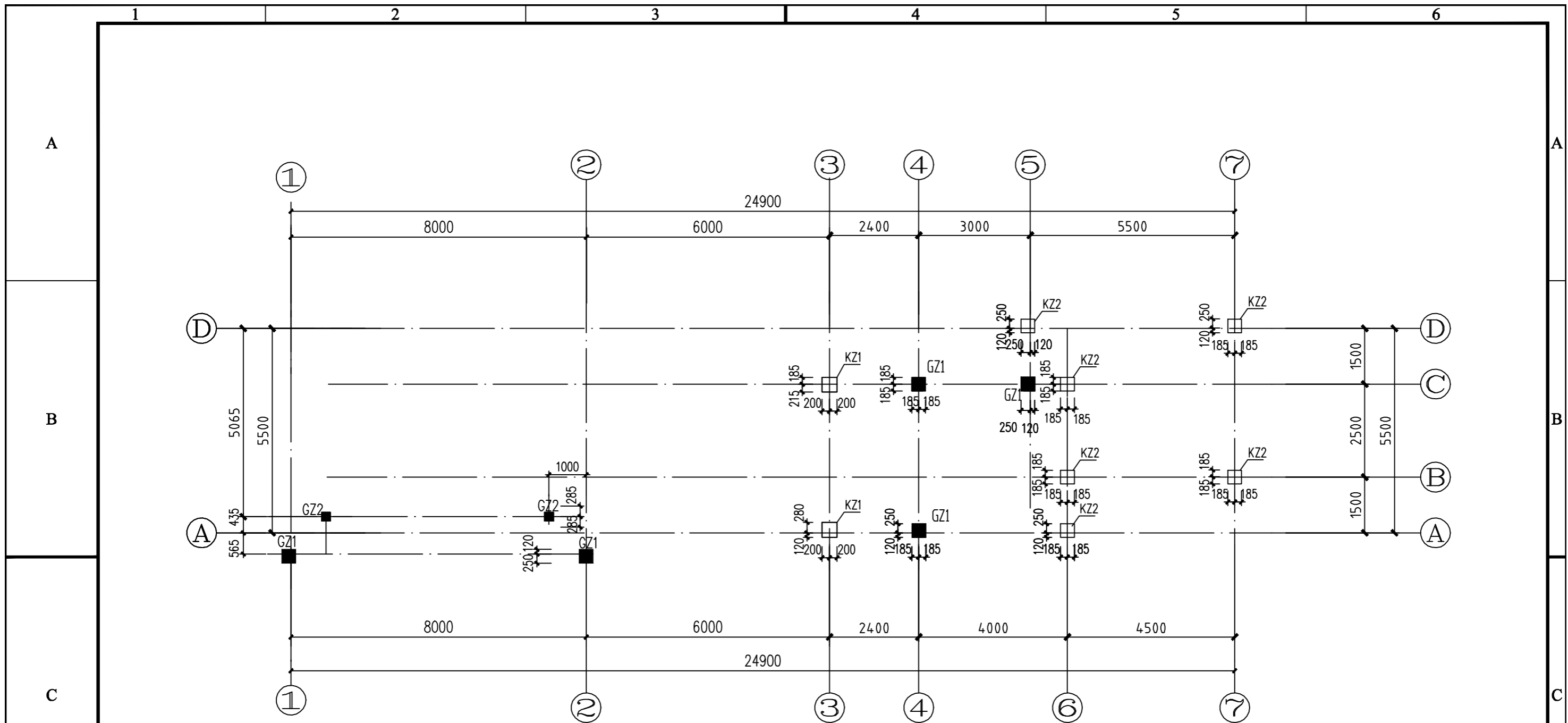
门卫室柱结构布置图 1:100
